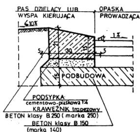
d) krawężnik trapezowy
