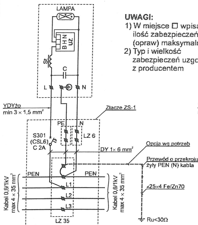
Schemat połączeń, przykład z ZS - 1 dla układu sieci TN-C
