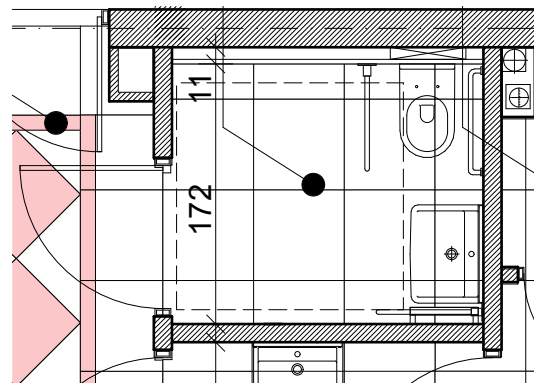
łazienka dla niepełnosprawnych
