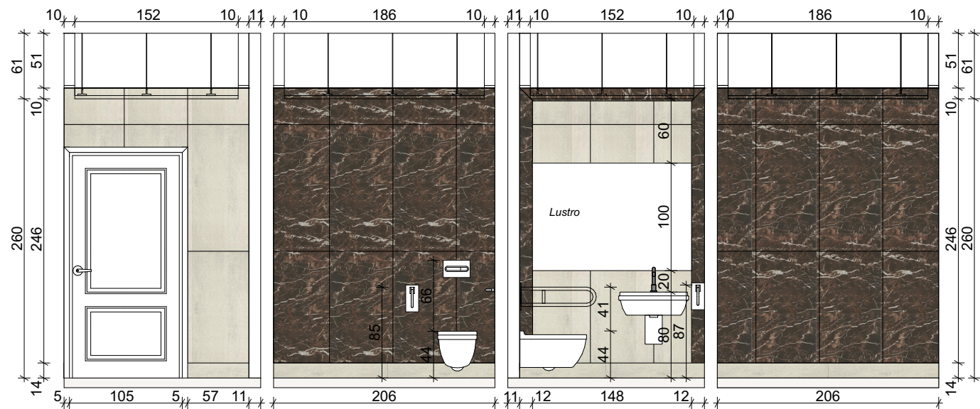
łazienka dla niepełnosprawnych
