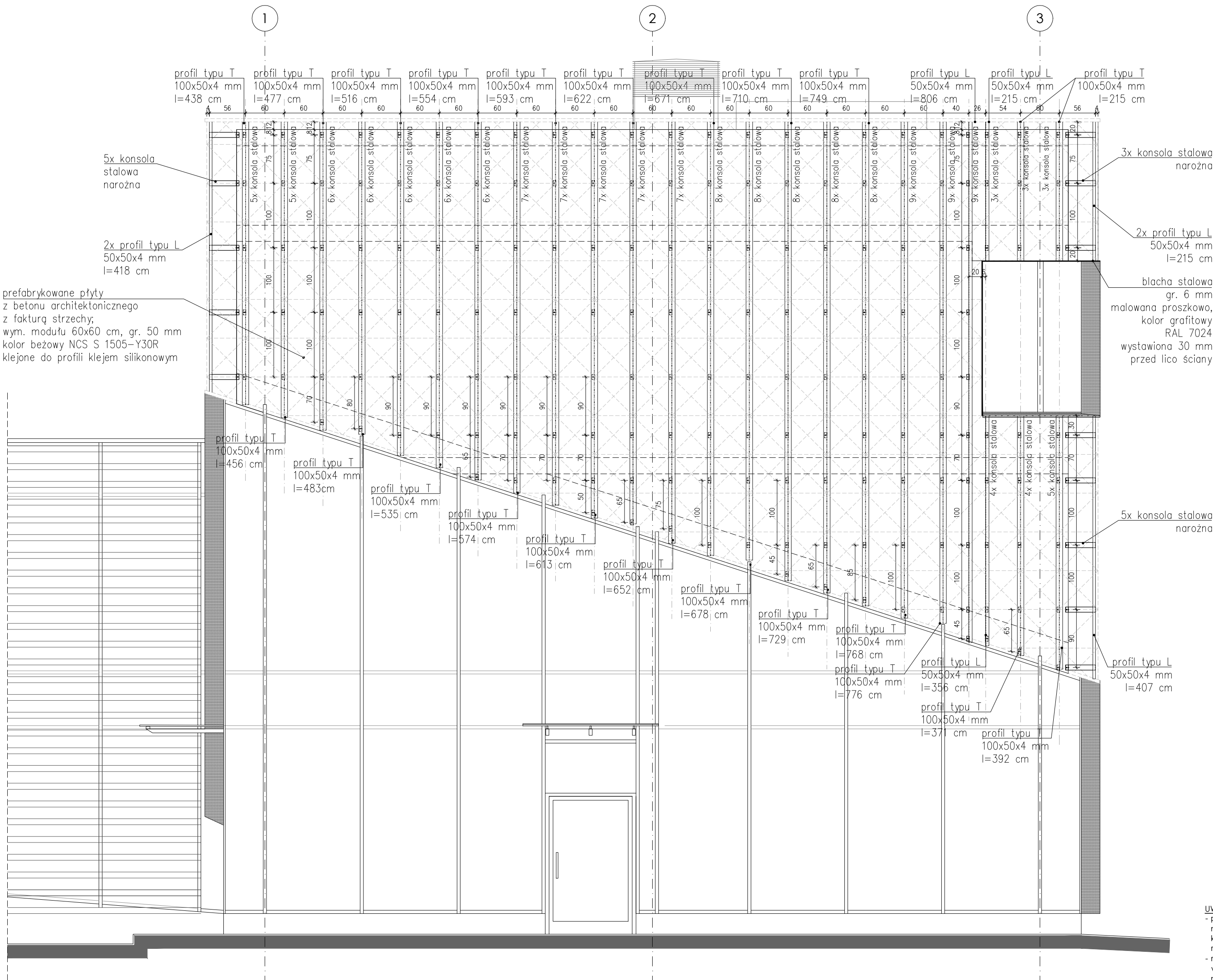
ELEWACJA ZACHODNIA
