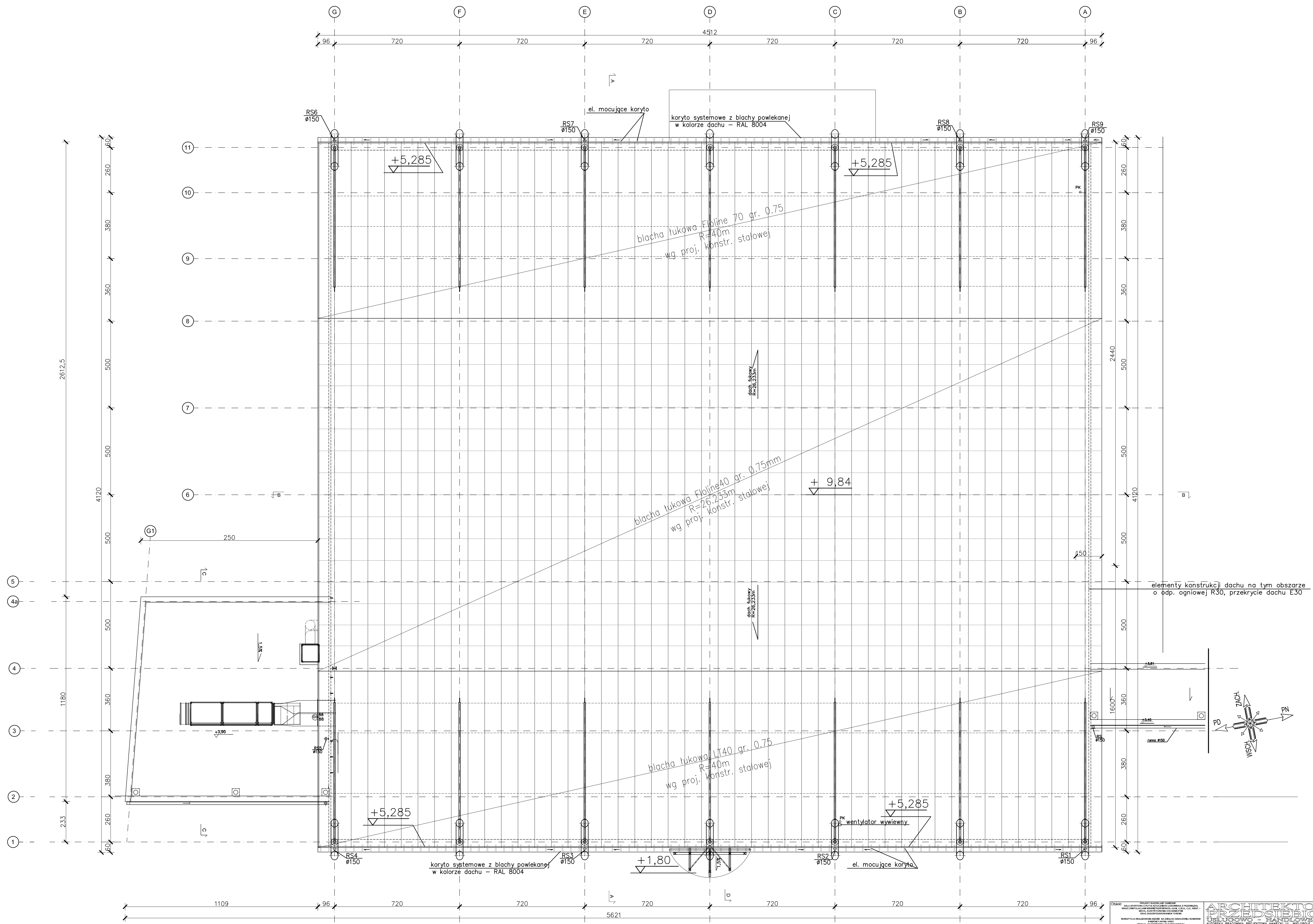
RZUT DACHU SKALA 1:100
