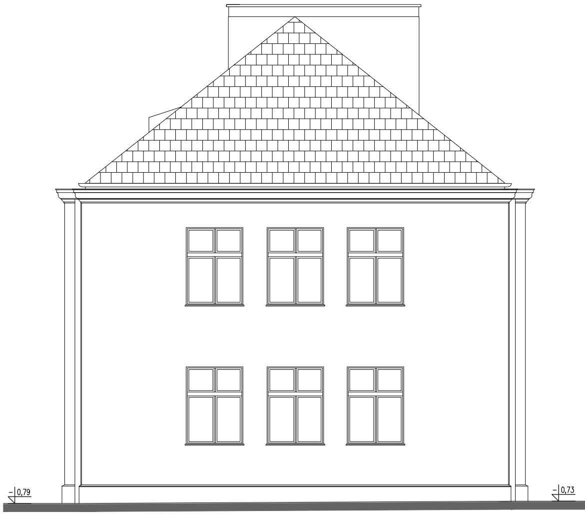
ELEWACJA POŁUDNIOWA
