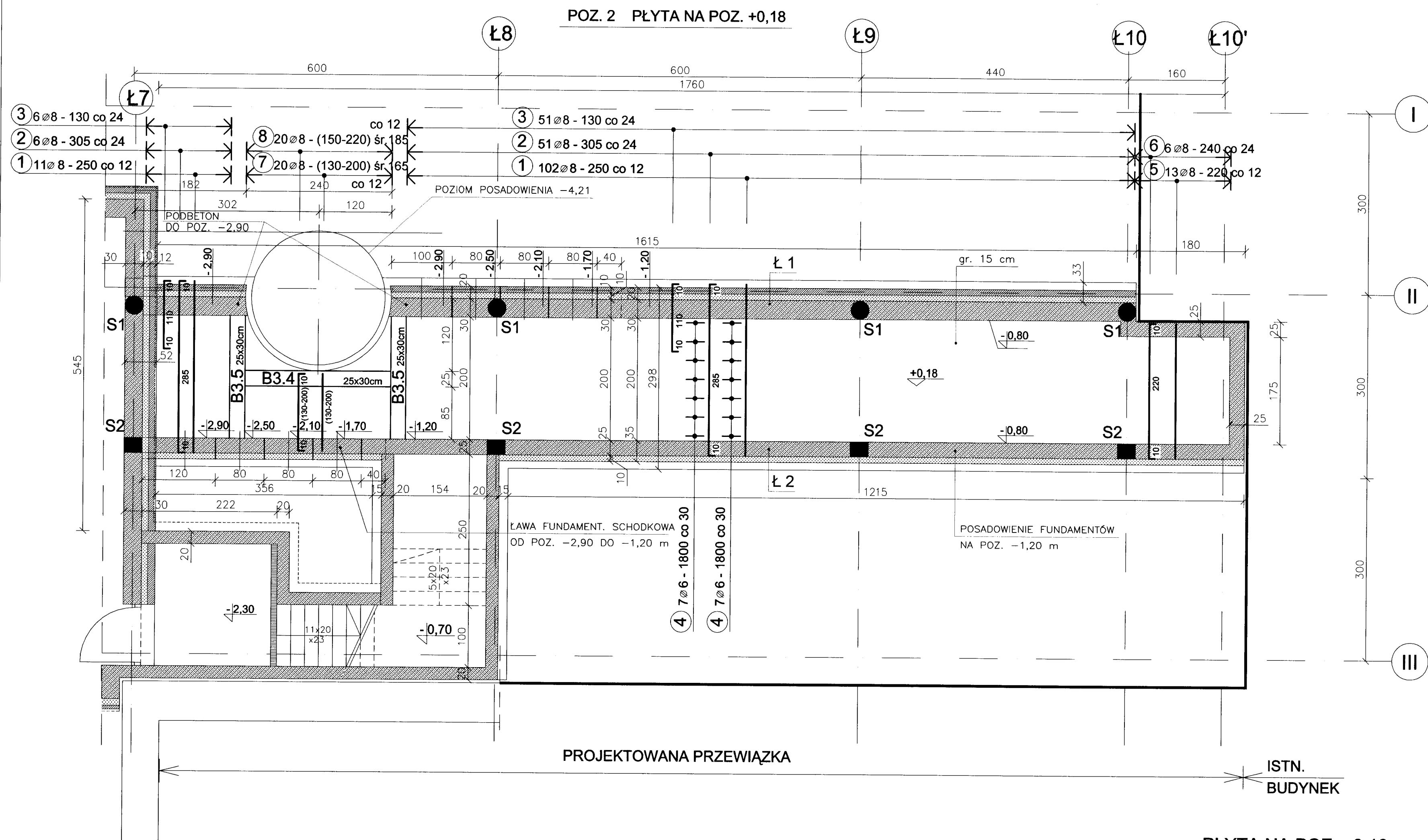
PŁYTA NA POZ. +0,18 skala 1:50
