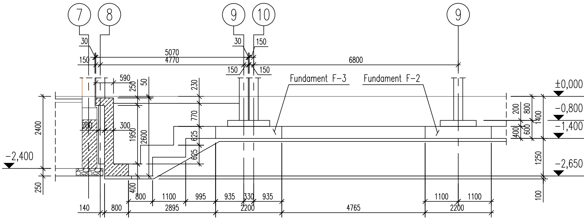
PRZEKRÓJ A-A 1:75
