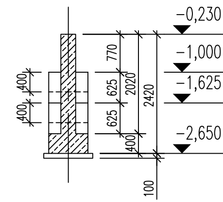
PRZEKRÓJ B-B 1:75
