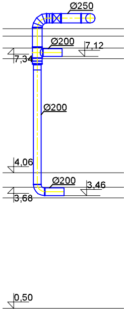
Schemat montażu pionu instalacji nawiewnej
