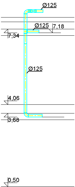
Schemat montażu pionu instalacji wyciągowej
