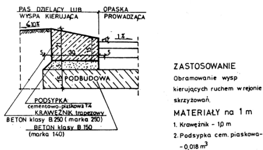
Rys. 1. Wymiarowanie krawężników
